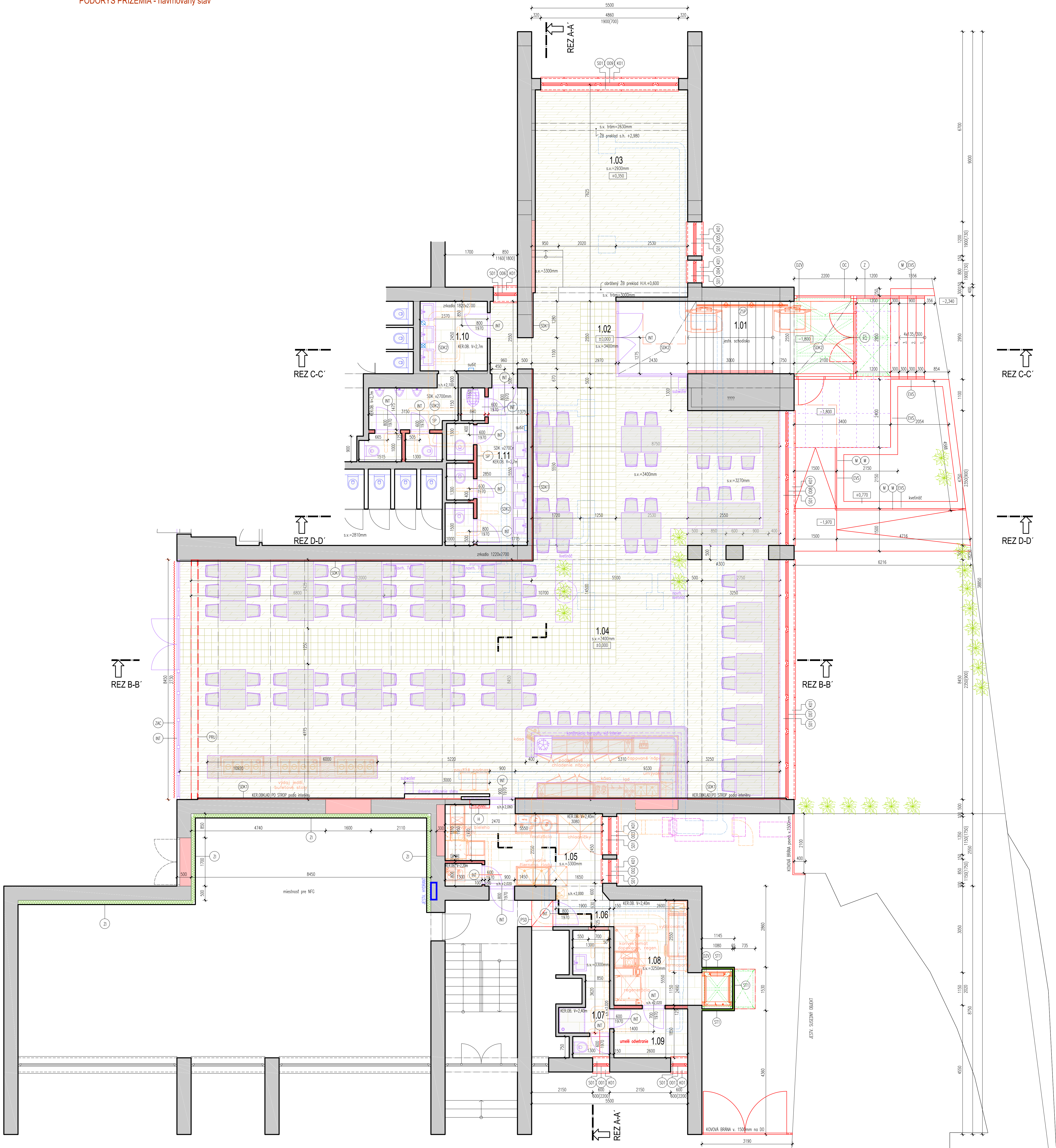
PÓDORYS PRÍZEMIA - navrhovaný stav
